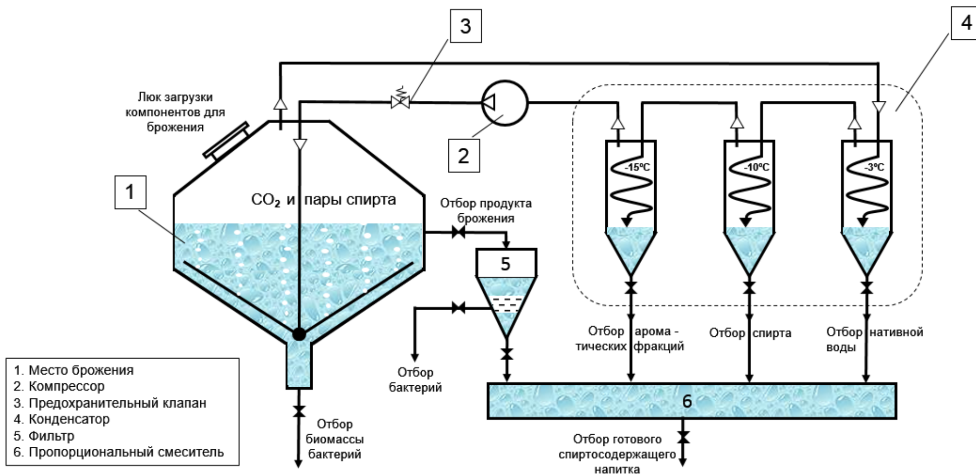
Фиг. 3 Пример реализации способа производства вина, пива и крепких алкогольных напитков
