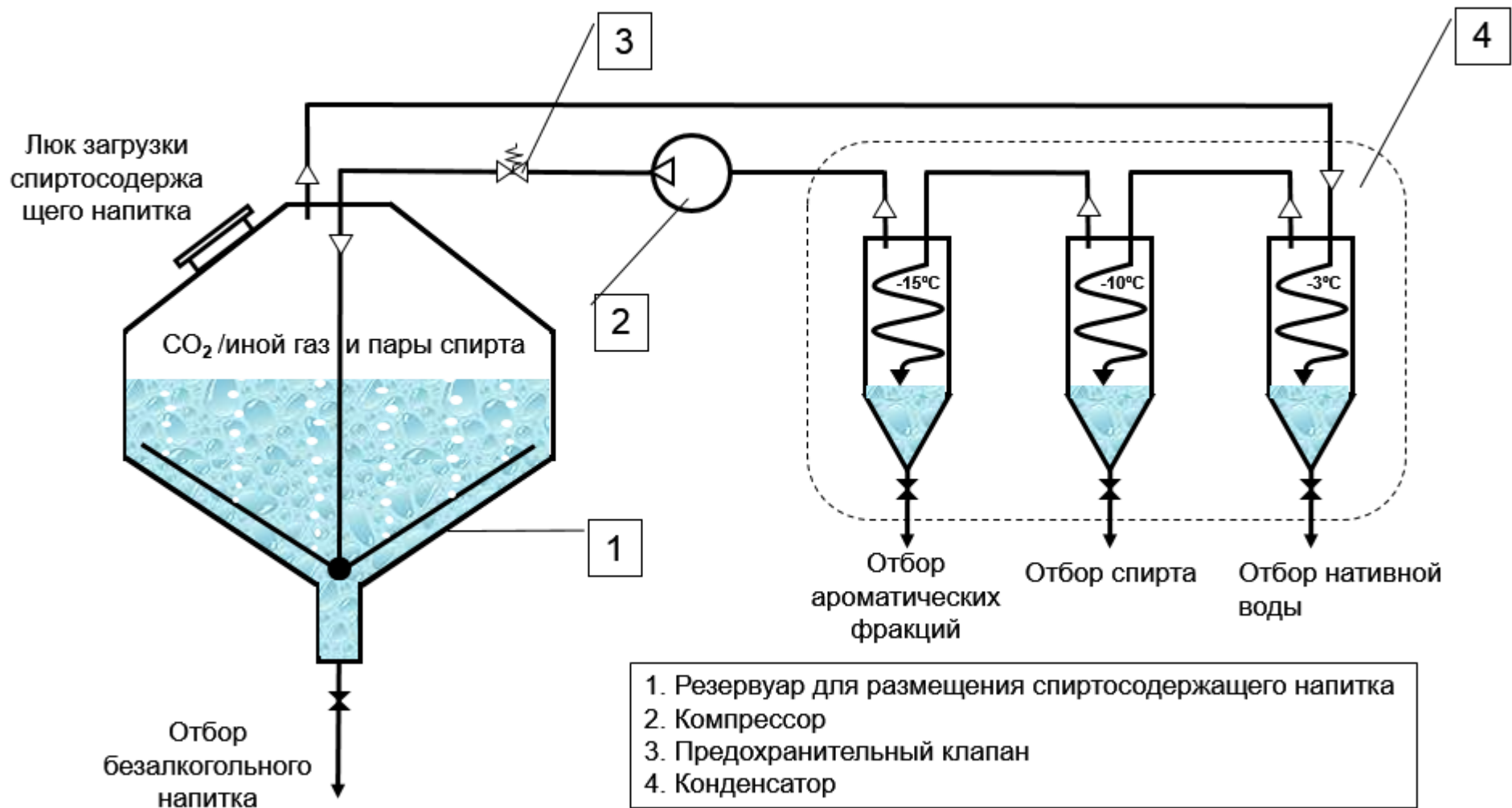
Фиг. 2 Пример реализации способа удаления спирта из спиртосодержащего напитка
